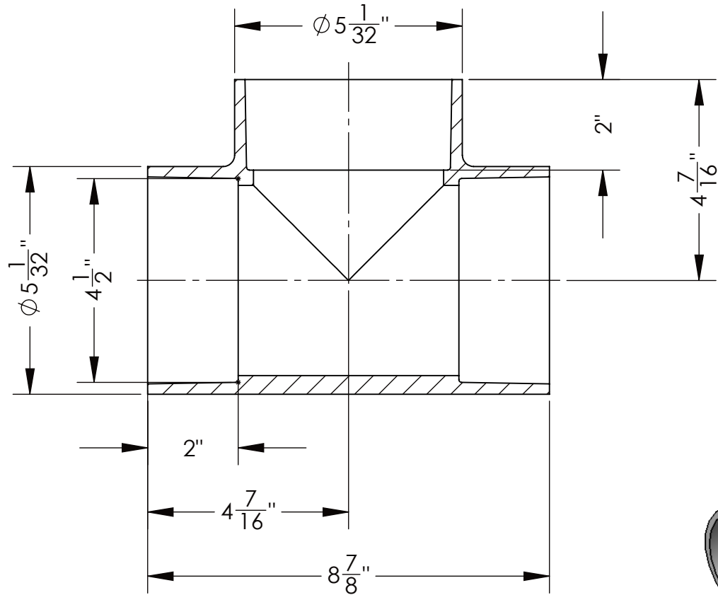
SECTION A-A
